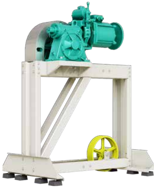
MR Dişlil Makine sehpası MR Gearbox Machine Frame Châssis de moteur geared MR Подлебедочная Рама СМП
