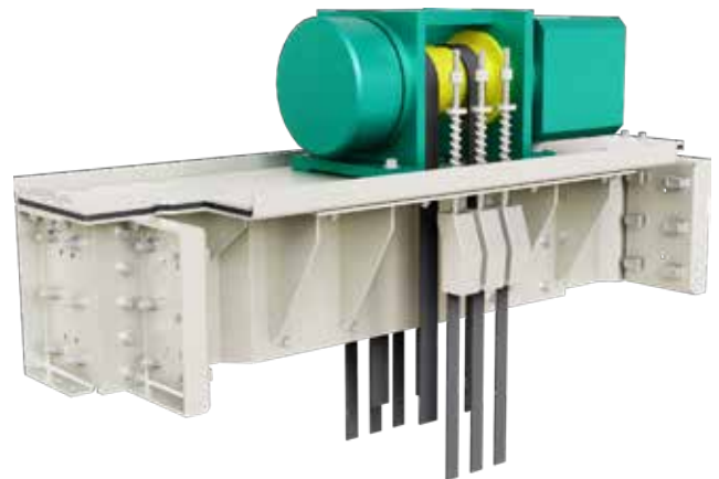
MRL Kayırlı Makine sehpası MRL Belt Machine Frame Châssis de moteur MRL à courroie Ленточная Рама СМП
