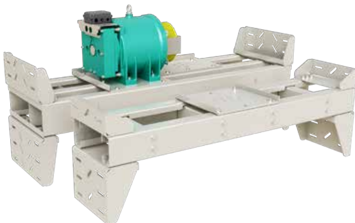
MRL - T Sistem Dişlisiz Makine Sehpası MRL - T System Gearless Machine Frame Châssis de moteur MRL gearless - Système T Подставка для безредукторного станка MRL-T System
