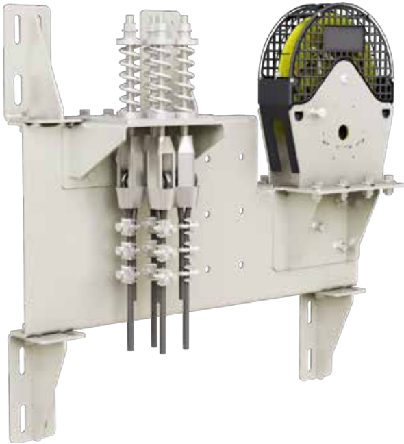
Fixpunt ve Regülatör Sehpası Fixpunt And Speed Governor Support Fixpunt et de régulateur Рама Fixpunt и Рама Регулятора
