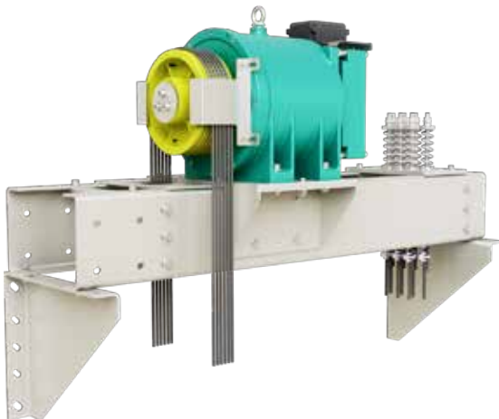
MRL Dişlisiz Makine Sehpası MRL - Gearless Machine Châssis de moteur MRL gearless Подлебедочная Рама БМП с настенным креплением
