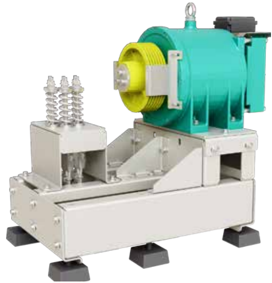
MR Dişlisiz Makine sehpası MR Gearless Machine Frame Châssis de moteur MR gearless Подлебедочная Рама БМП
